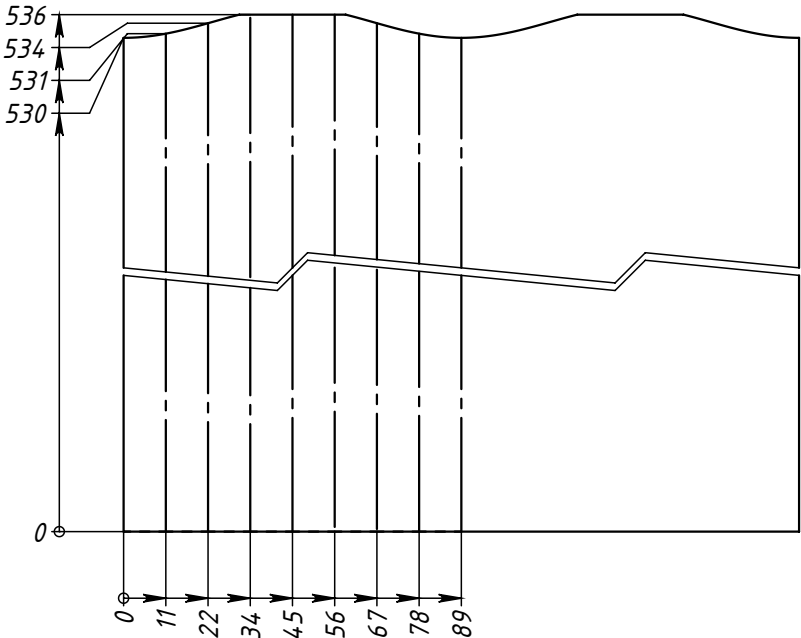
Поз.3 (Труба) развертка 1:2
